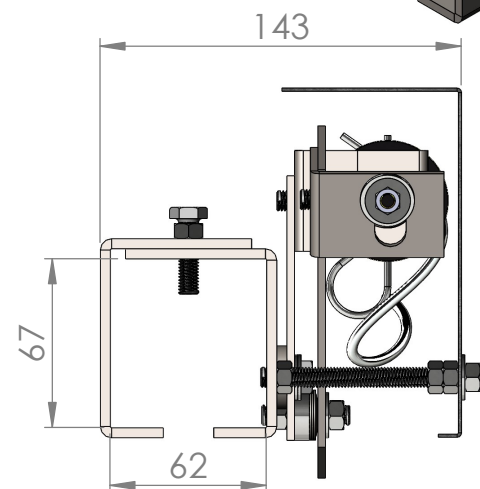
Pince pour Rail type 5
